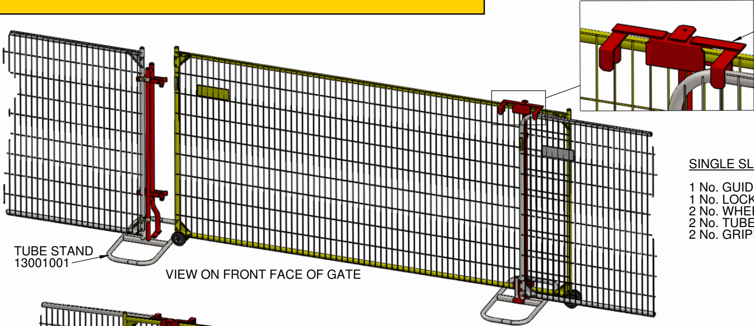
GRIPPER COUPLER 08551320
